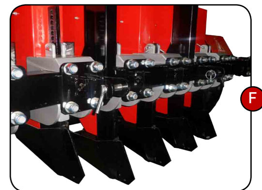
F. Rejas de siembra regulable en altura.
