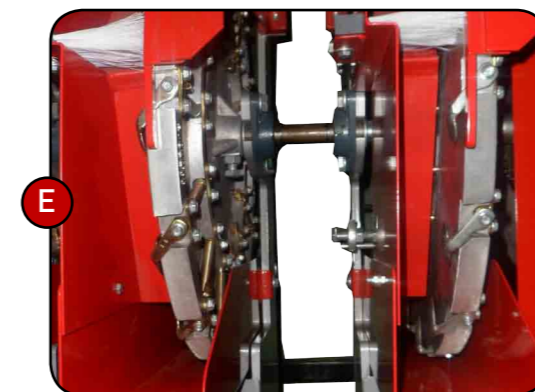
E. Cuerpos de siembra.
